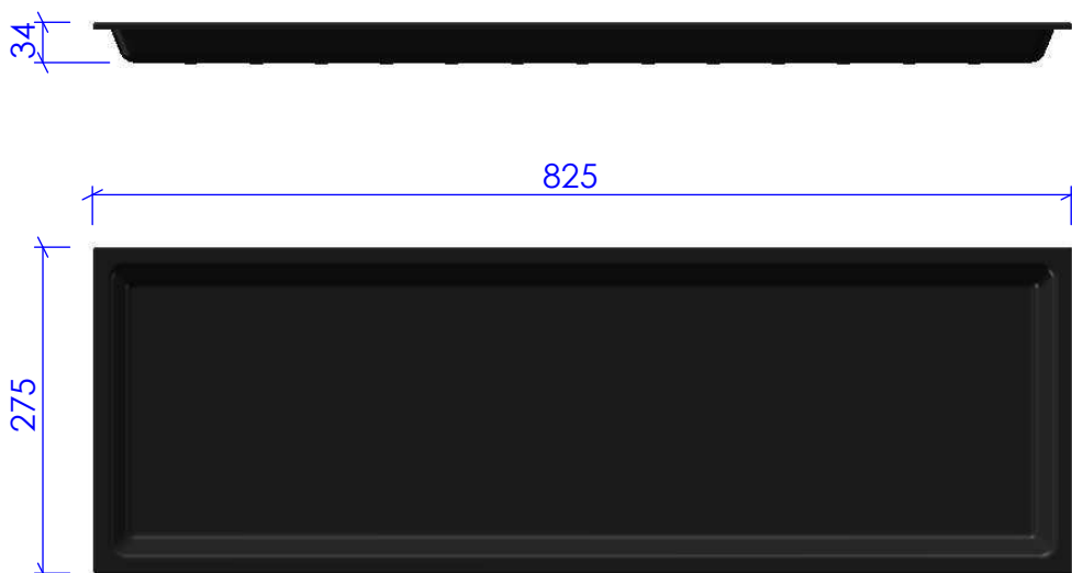
Tabuleiro 825x275x34mm
