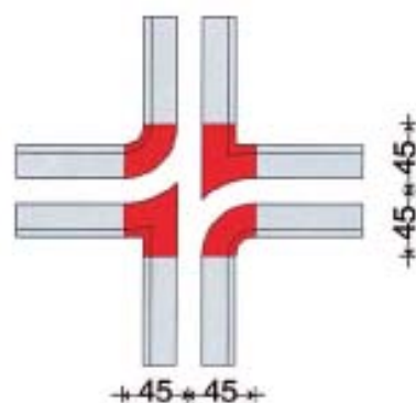
Agulha de Quatro Vias
